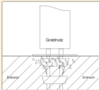
■ Pfahlgründung / Erdfix
