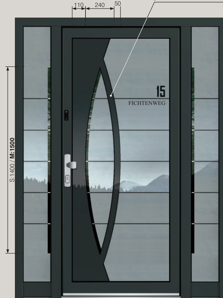
ASS 1865 Ganzglasfüllung Glas ESG mittig Alu Applikationen im LZR Zubehör Glasmotiv MS 6730 + Hausnummer HFG GA 190 S P Farbe RAL 7016 matt Alu Appl. im LZR RAL 7016 matt Seitenteil ST 01 / WG / 400 Glasmotiv MS 6730/S Option: Fingerscan
